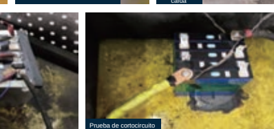
Prueba de cortocircuito
